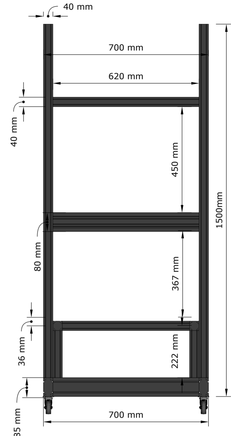
VISTA FRONTAL ESC: 1/50
