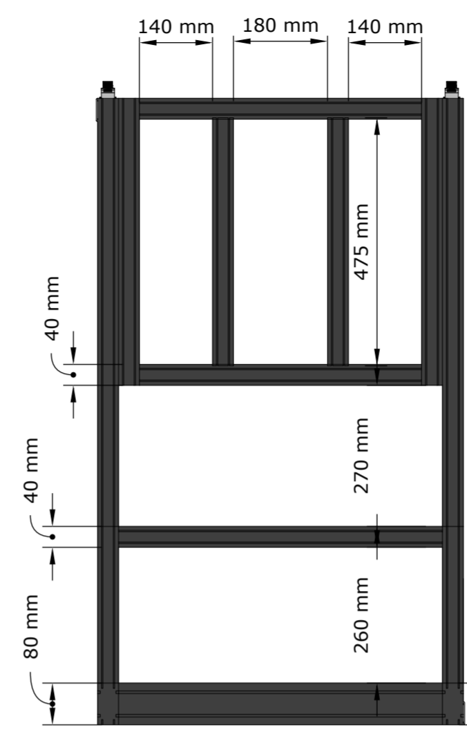
VISTA SUPERIOR ESC: 1/50
