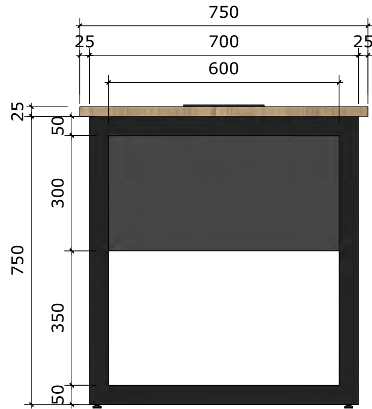
VISTA LATERAL ESC. 1:10
