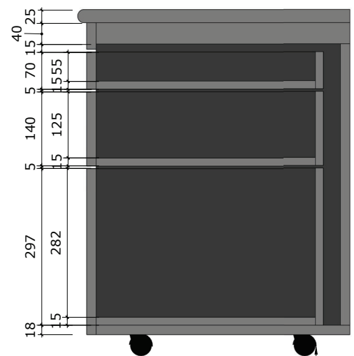
CORTE BB ESC. 1:5
